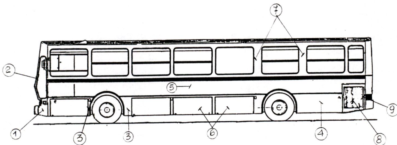
FIG. 3 - LATO SINISTRO
